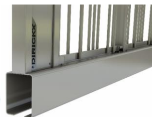
Poutre 160 x 220 mm pour les passages de 8 m à 10 m (Tôle de 6 m à 7,50 m)
